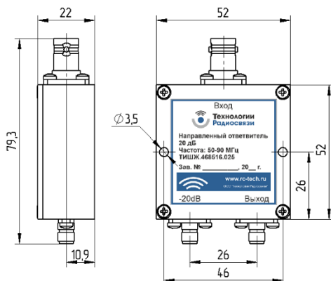
Рисунок 1 – Общий вид изделия.
